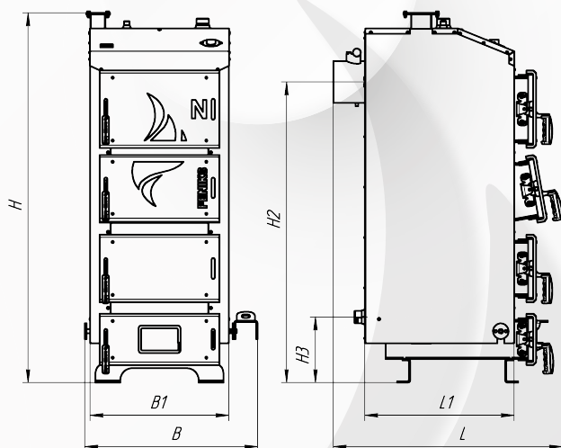
Рисунок 1 – Позначення габаритів котла
